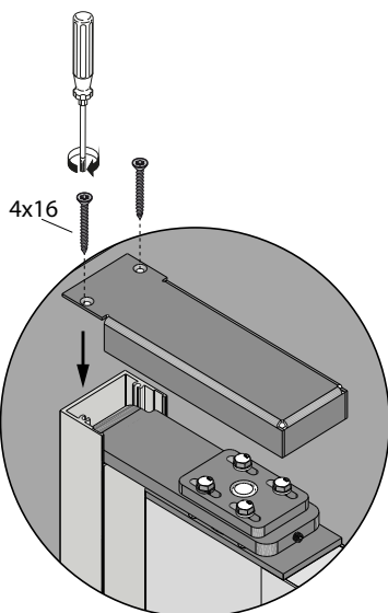
PUERTA CON MARCO
